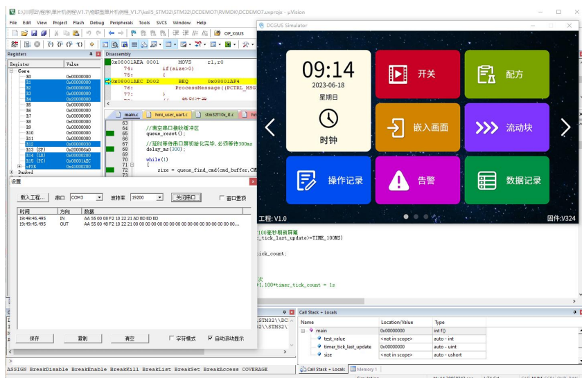
图 8-3Keil 开发环境与“HMI 模拟器”绑定调试
