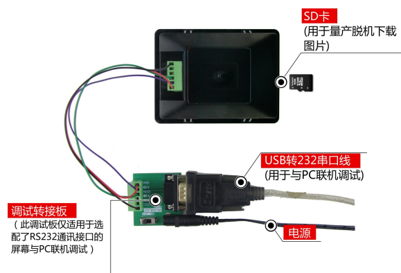
图 1-4 RS232 调试工具图
