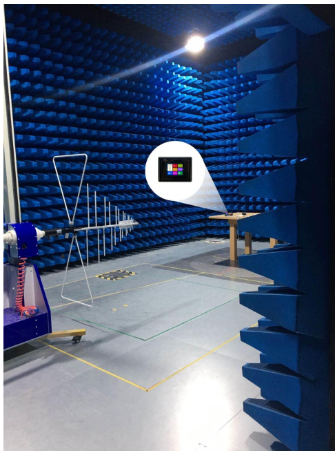
图 6-5 辐射测试图
