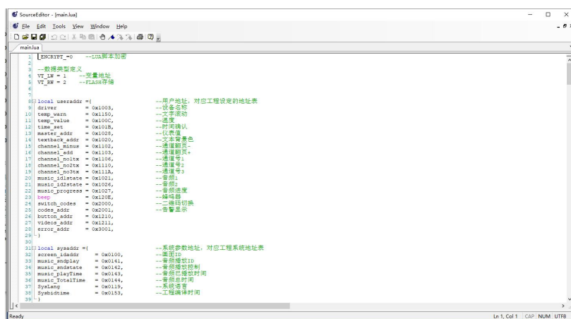
图 10-2LUA 脚本编辑器
