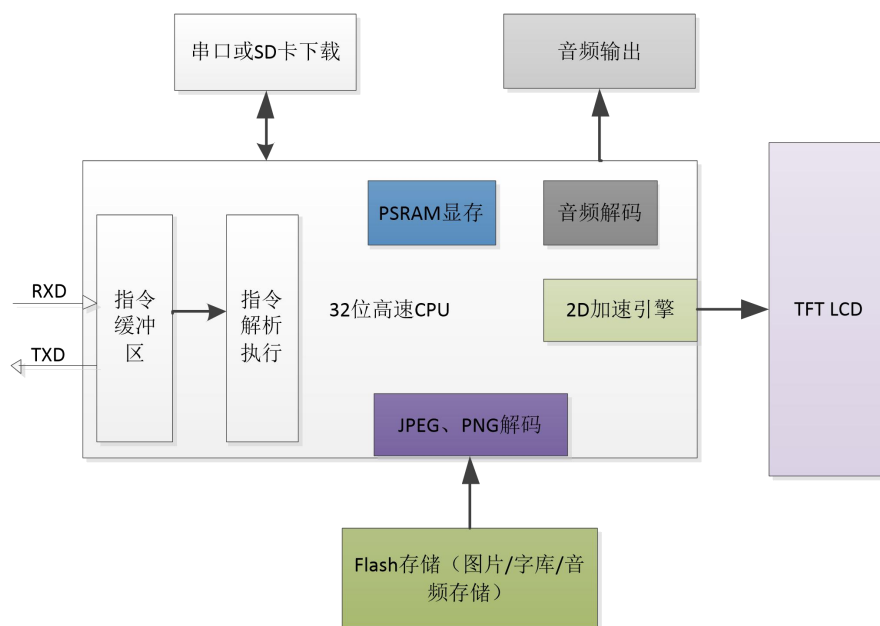
图 3-1 DN 系列串口屏内部结构图
