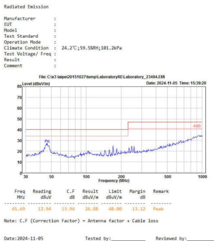
图 6-7 辐射测试垂直方向
