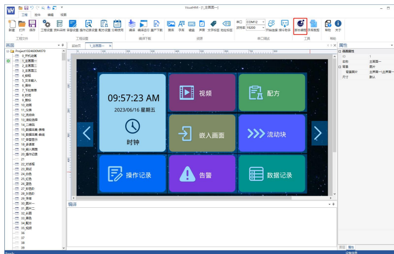
图 10-1LUA 脚本编程
