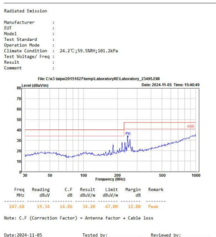
图 6-6 辐射测试水平方向
